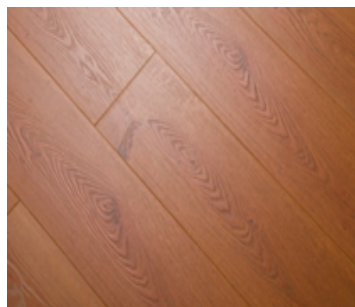
LR04
